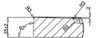
B SCALE 0,5
